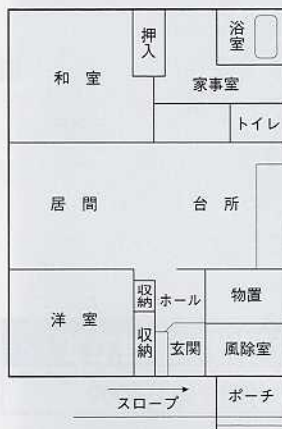
塚Ⅱ住宅 木造平屋建
